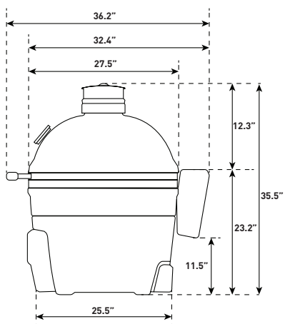
ZIJAAANZICHT
